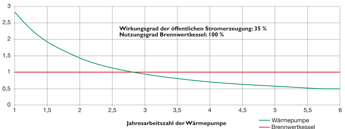
Primärenergieeinsatz (kWh) für 1 kWh Heizwärme
